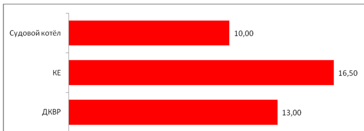
Рисунок 2.15 – Суммарная установленная мощность котлов в группе котельных мощностью - 20 Гкал/ч
