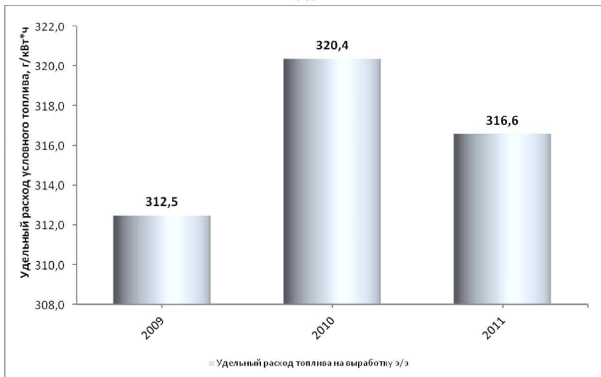
Рисунок 2.12 - Изменение удельного расхода условного топлива на отпуск электрической энергии Архангельской ТЭЦ
