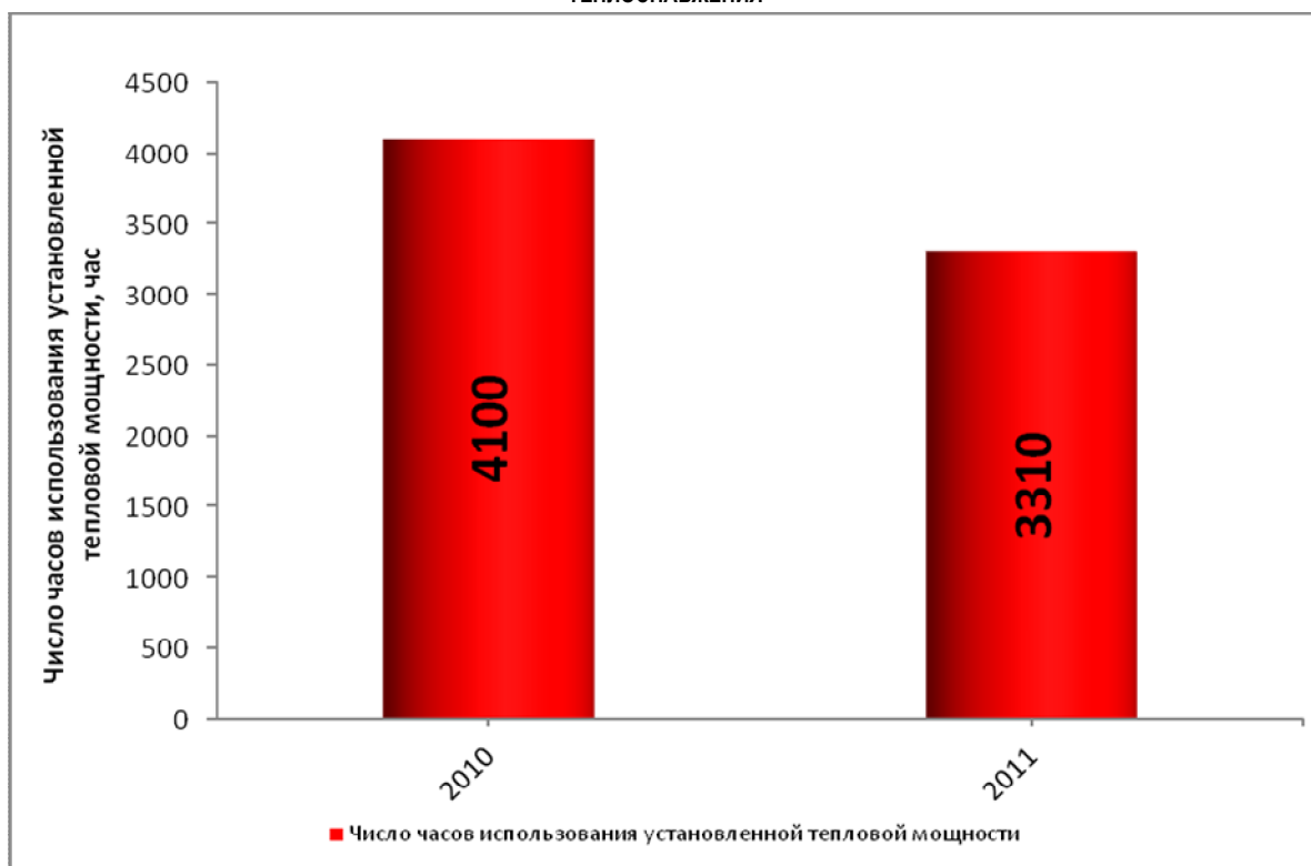
Рисунок 2.8 – Среднегодовая загрузка тепловой мощности турбоагрегатов Архангельской ТЭЦ
