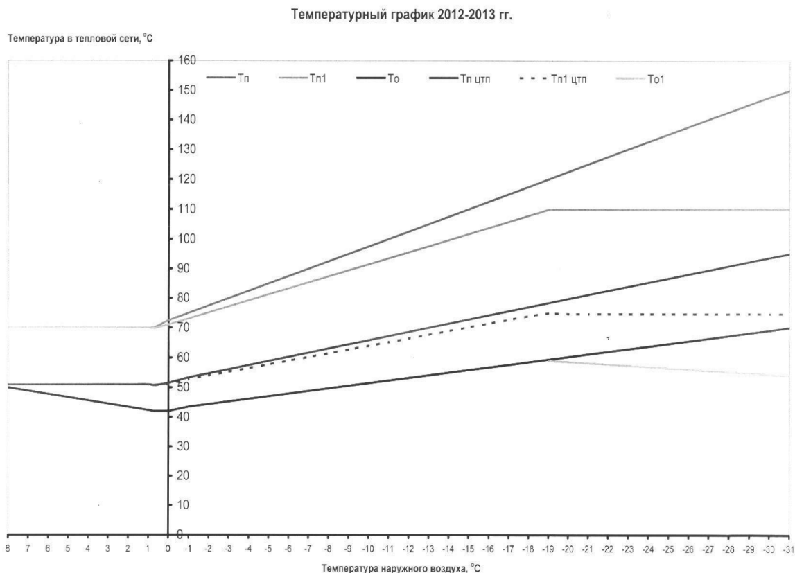
Рисунок 3.6 – Температурный график отпуская тепловой энергии Архангельская ТЭЦ
